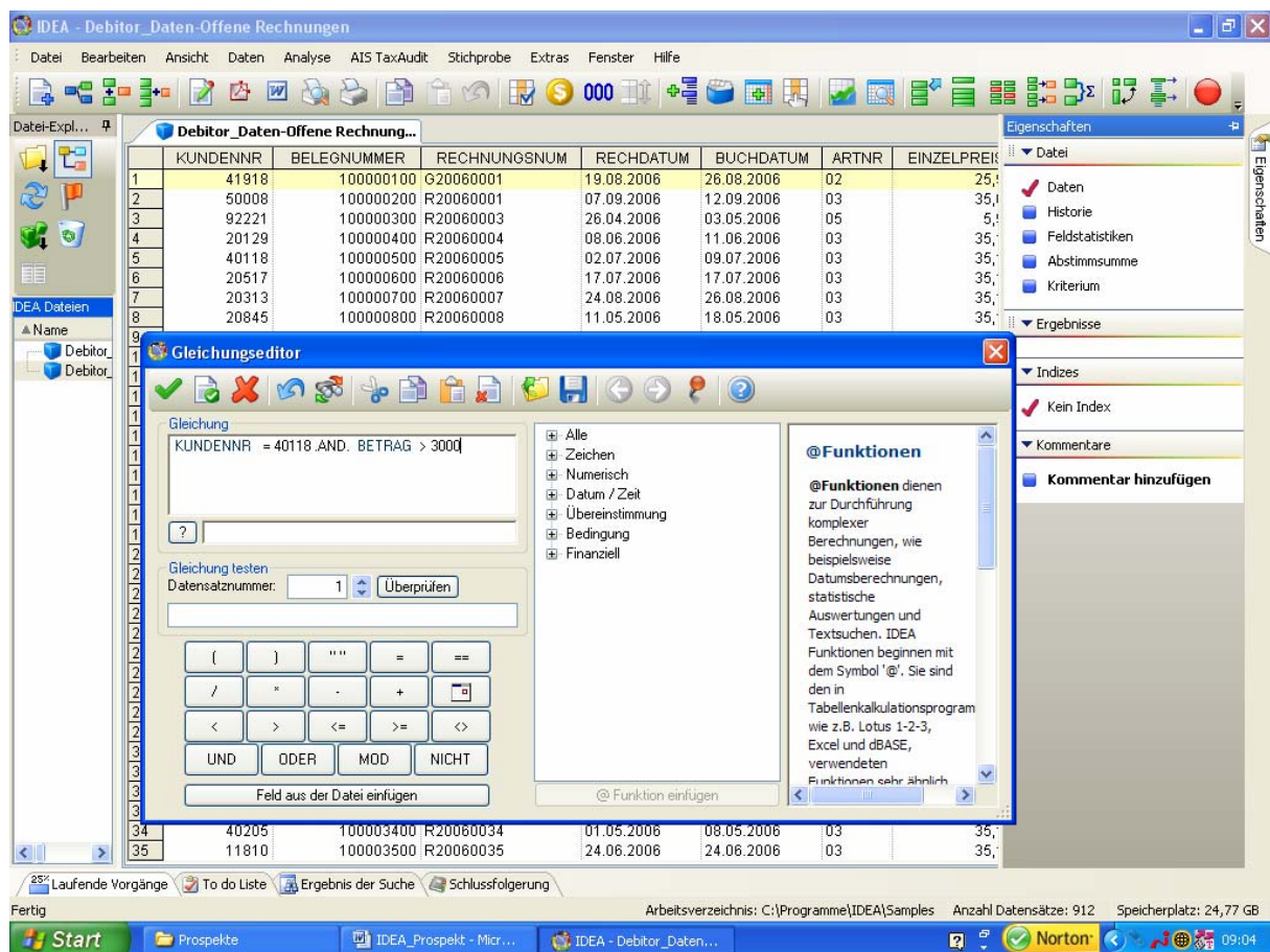
Abb. 2 Abfrage Ihres Datenbestandes nach beliebigen Kriterien.
